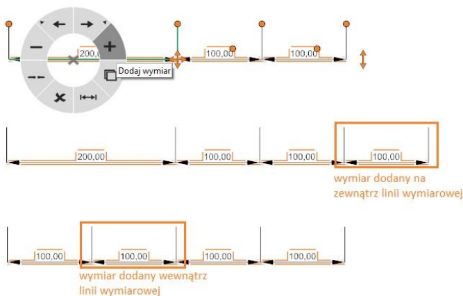
Rys. 233 – dodawanie nowego odcinka linii wymiarowej – na zewnątrz i wewnątrz
