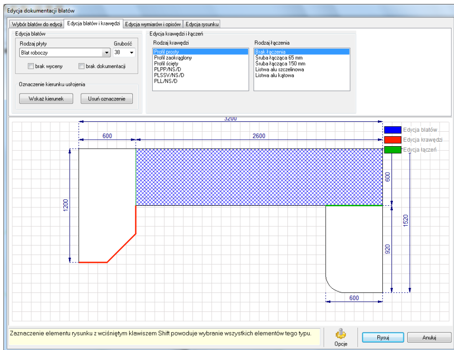
Rys. 245 - okno „Edytora blatów” – podgląd blatów, krawędzi i łączeń
