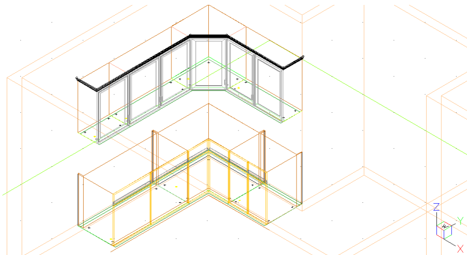
Rys. 265 – wyrysowanie w oparciu o ścieżkę listwy górnej
