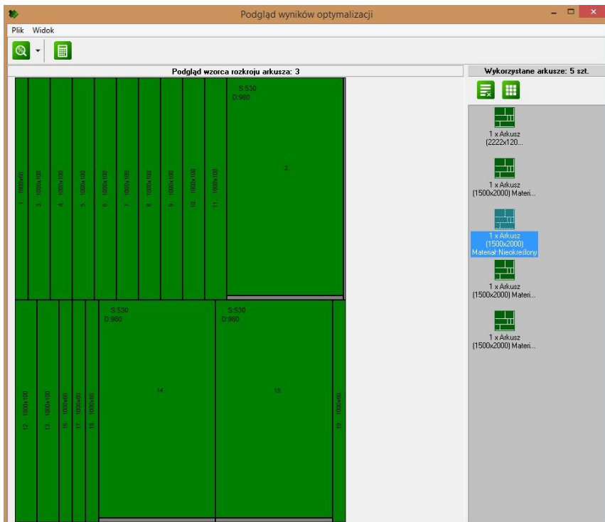
Rys. 521 – przykładowy wzorec rozkroju formatek szafy wewnętrzej w programie CAD Rozkrój v. 4
