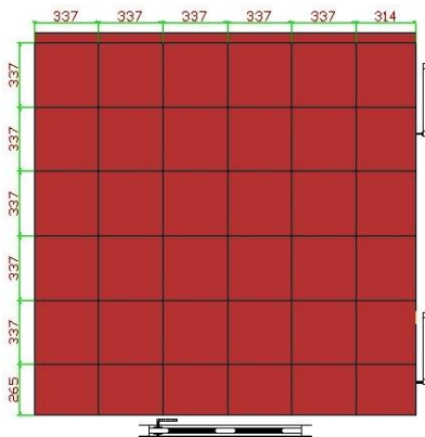
Rys. 405 - zwymiarowany kład płytek
