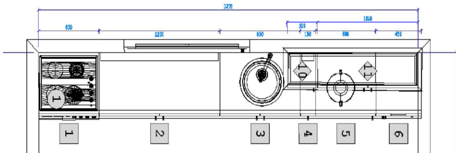
Rys. 312 – rzut z dokumentacji w środowisku IntelliCAD
