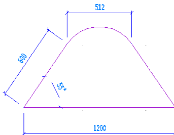
Rys. 148 - trapez zwieńczony łukiem
