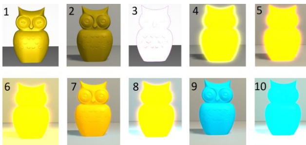
Rys. 463 – ten sam obiekt z różnymi ustawieniami podświetleń i emisji, w różnym oświetleniu (tylko bezpośrednie lub globalne)
