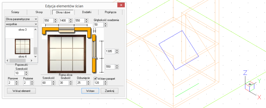
Rys. 132 - wstawianie okna w skos - okno edycji i podgląd w środkowisku
